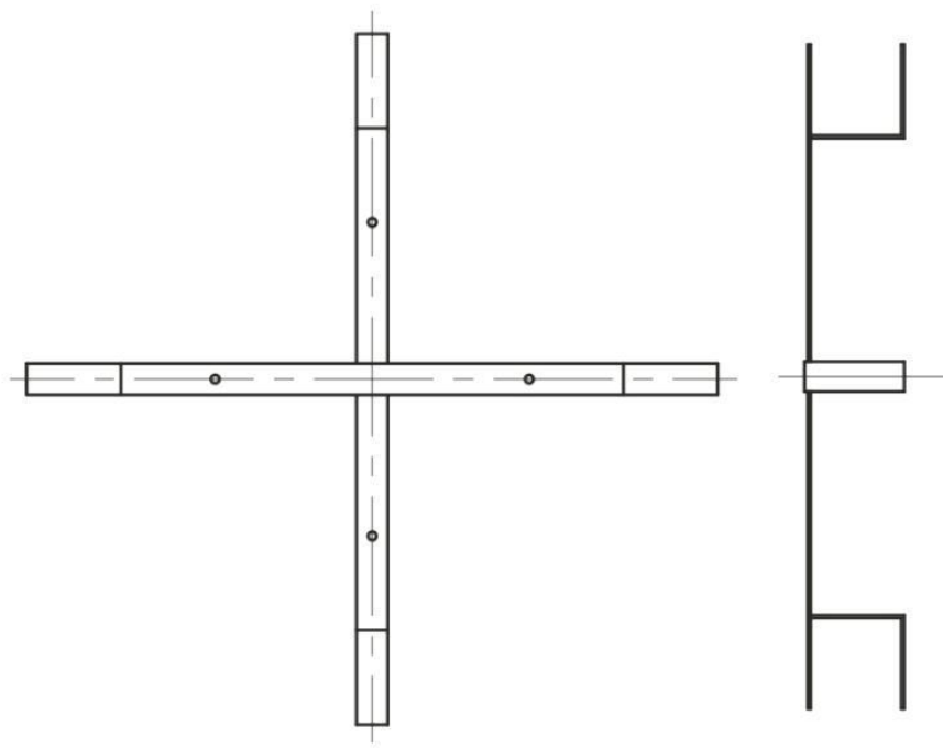
Spare Cable Rack for OPGW OPGW光缆余缆架
